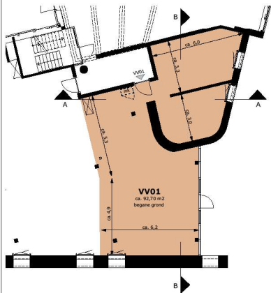
Begane grond
