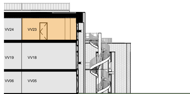
Doorsnede B-B
