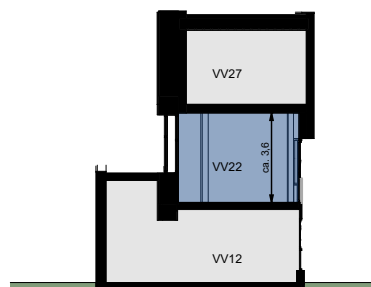
Doorsnede B-B
