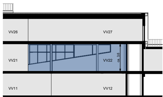
Doorsnede A-A
