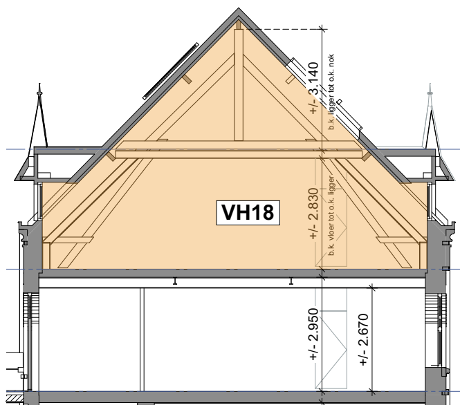
Doorsnede A-A
