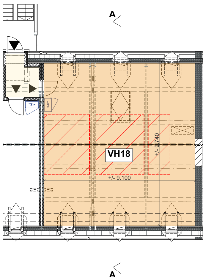
Derde verdieping
