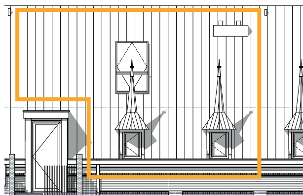
Voorgevel
