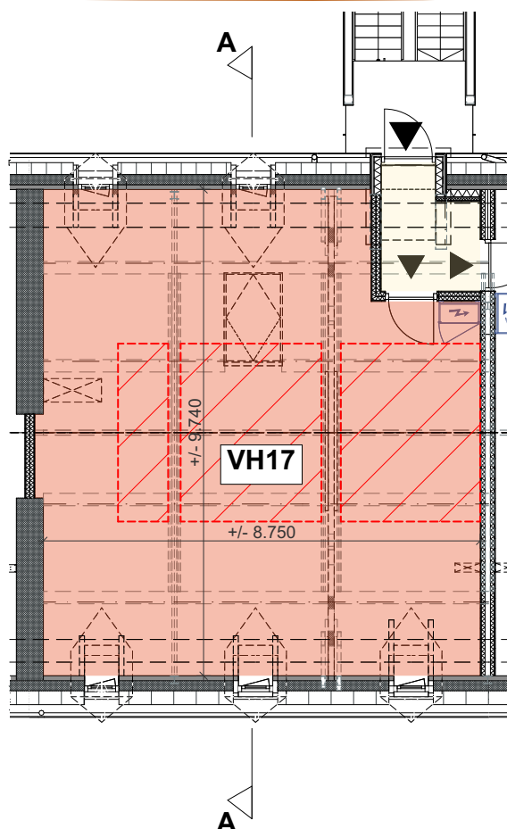
Derde verdieping
