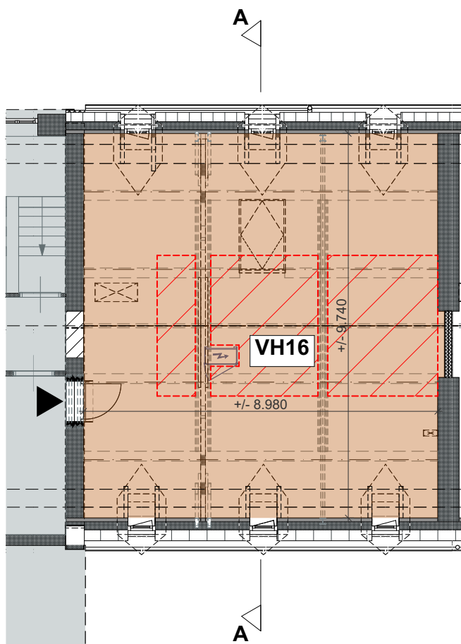
Derde verdieping
