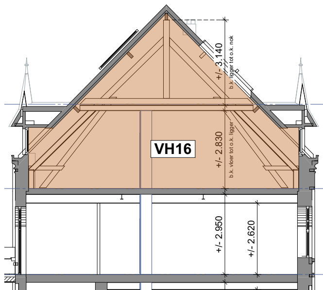
Doorsnede A-A
