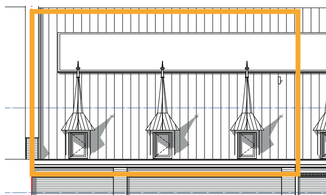
Achtergevel
