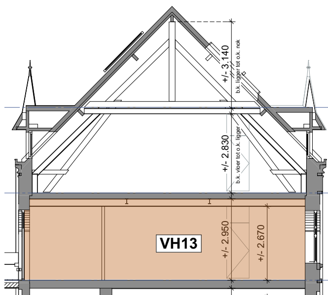
Doorsnede A-A
