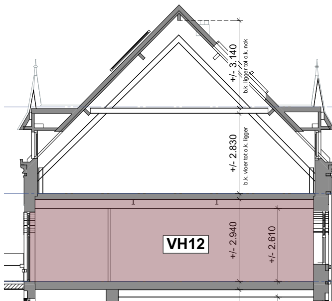
Doorsnede A-A
