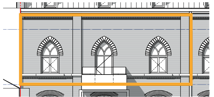
Achtergevel
