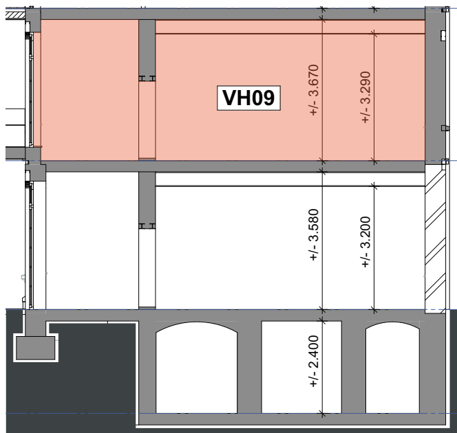
Doorsnede A-A
