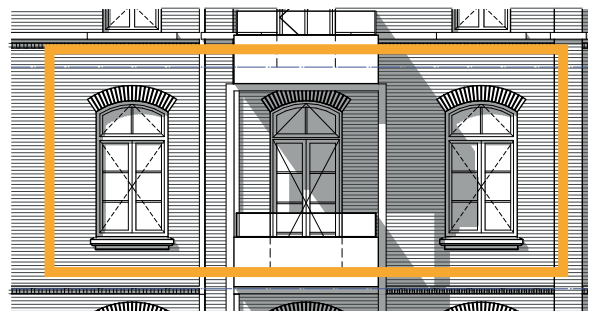
Achtergevel
