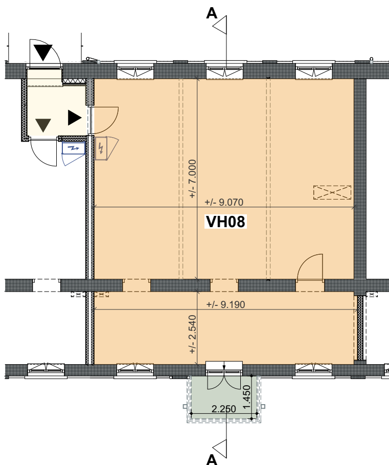
Eerste verdieping
