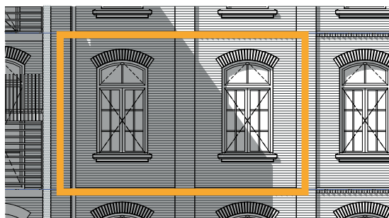
Voorgevel
