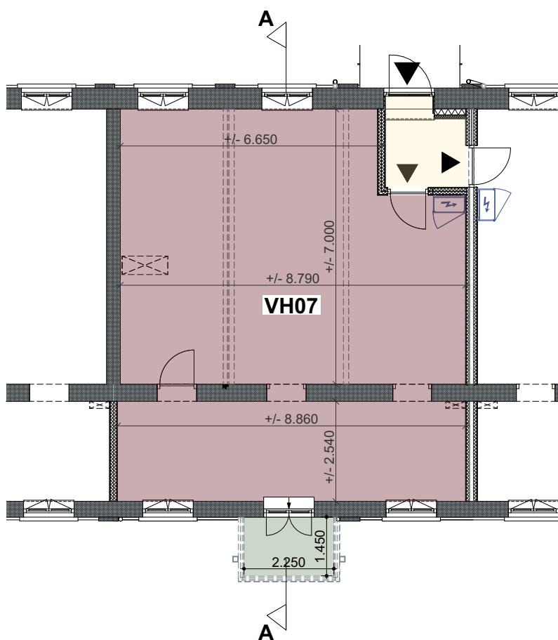
Eerste verdieping
