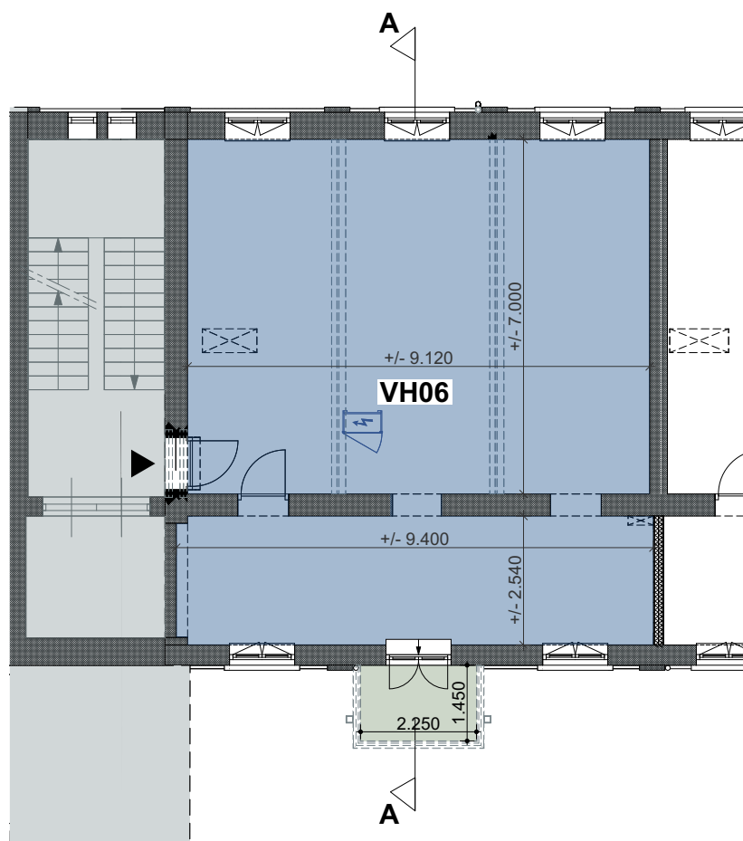
Eerste verdieping
