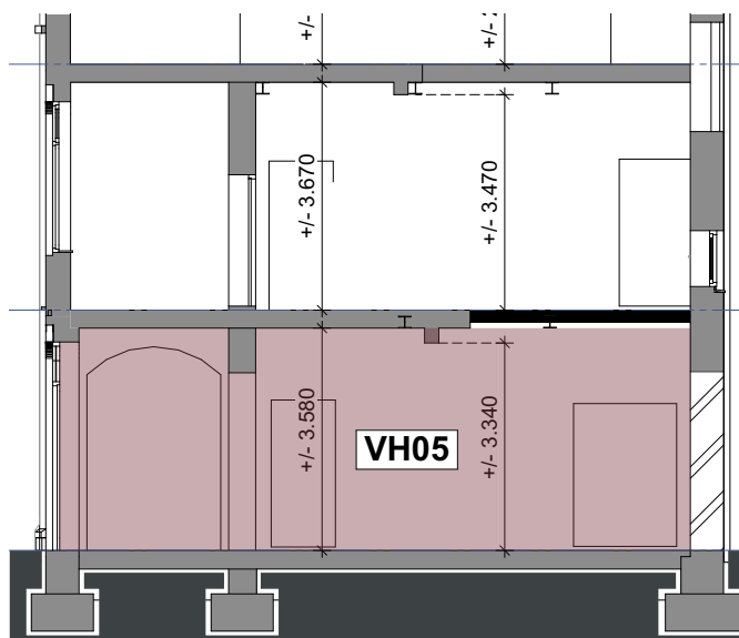
Doorsnede A-A
