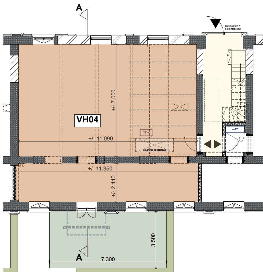
Begane grond
