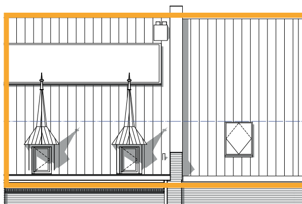
Achtergevel
