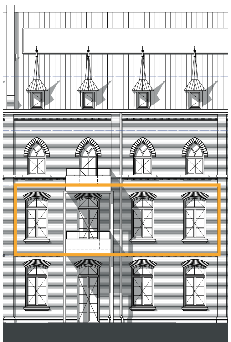
Achtergevel
