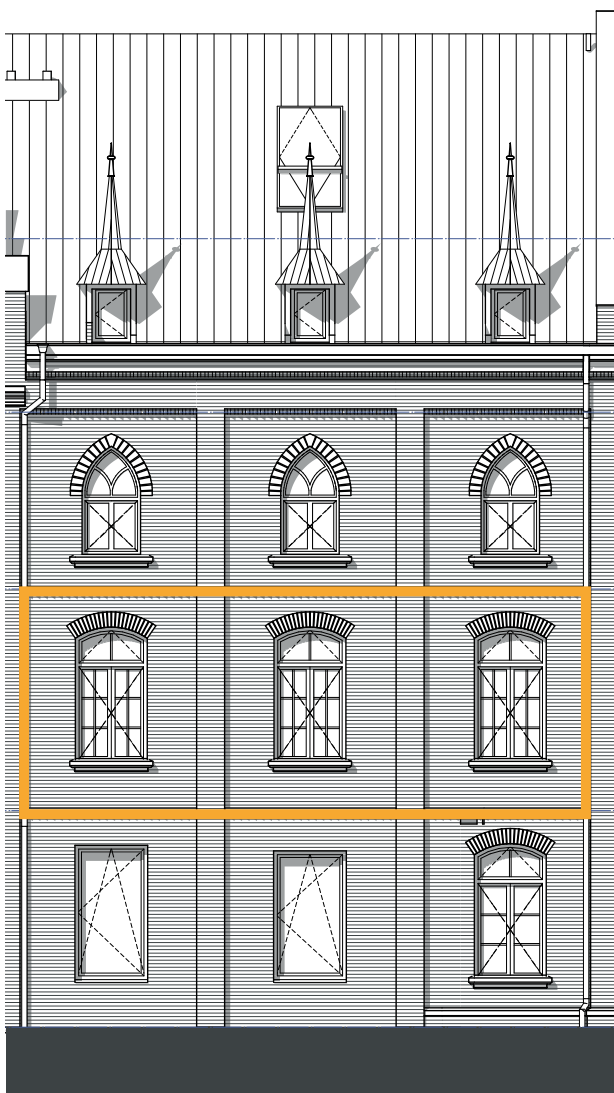
Voorgevel
