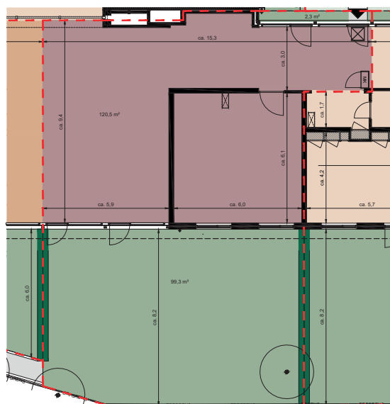
Begane grond
