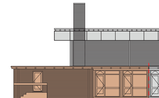
Zuid gevel
