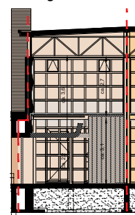
Doorsnede B-B
