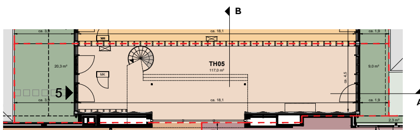
Begane grond
