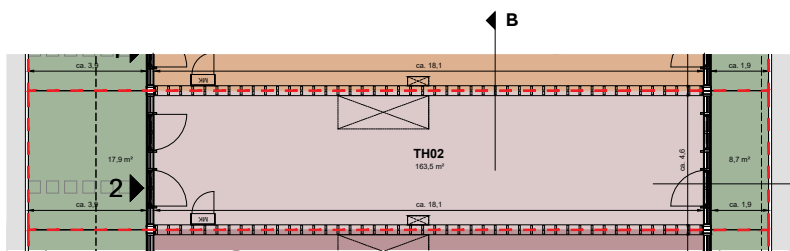
Begane grond
