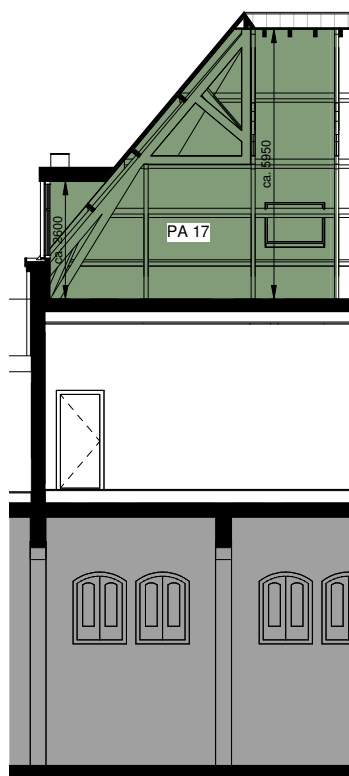
Doorsnede a
