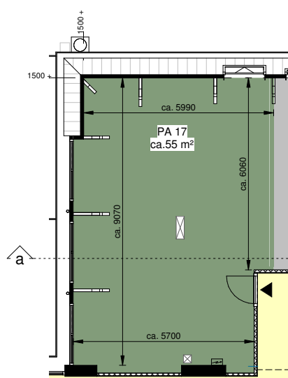
Tweede verdieping
