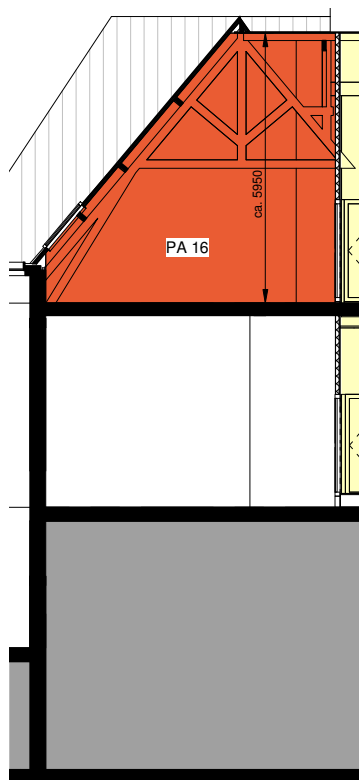
Doorsnede a
