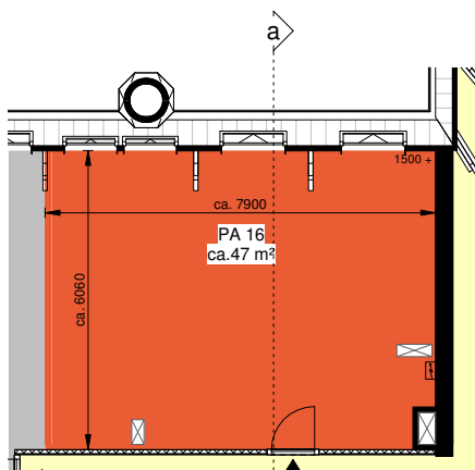
Tweede verdieping
