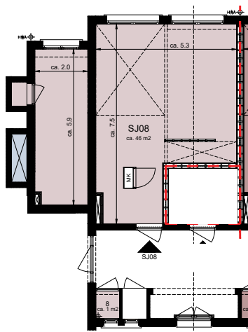
1e verdieping
