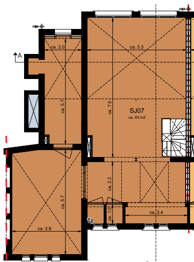
2e verdieping
