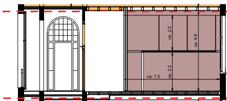
Doorsnede
