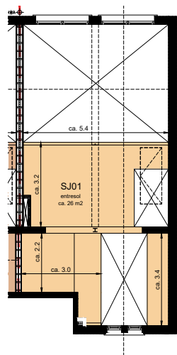
2e verdieping entresol
