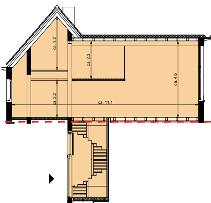
Doorsnede
