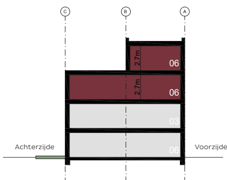
Doorsnede dwars
