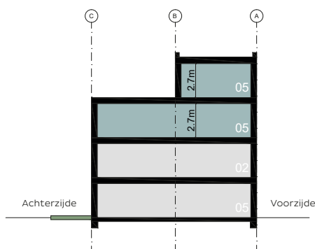
Doorsnede dwars
