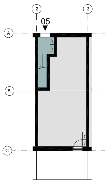
Begane grond
