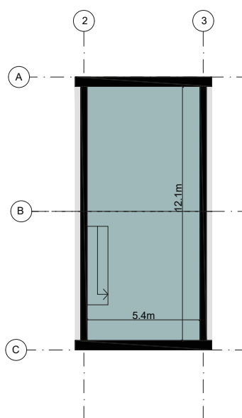
Tweede verdieping
