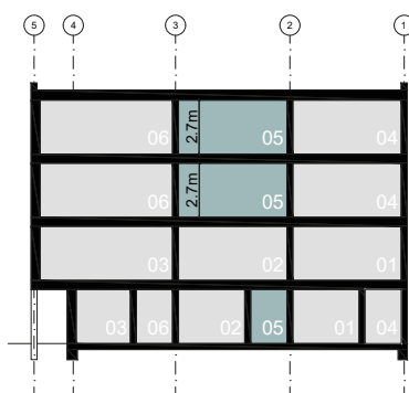
Doorsnede, straatgevel
