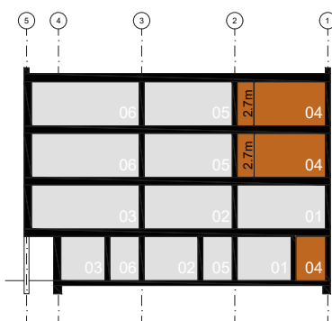
Doorsnede, straatgevel
