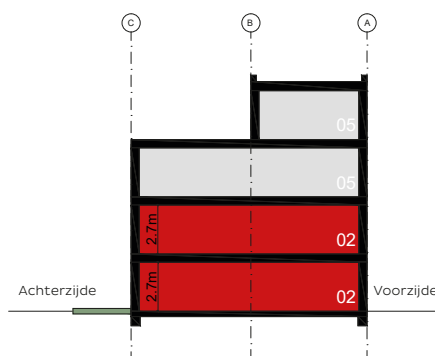
Doorsnede dwars
