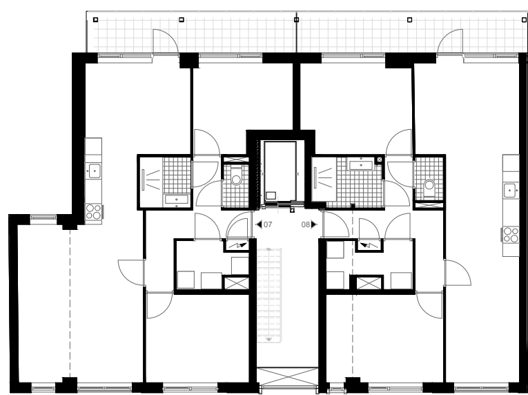
Derde verdieping
