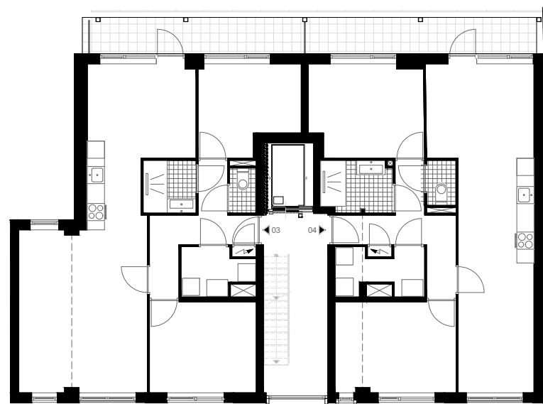
Eerste verdieping
