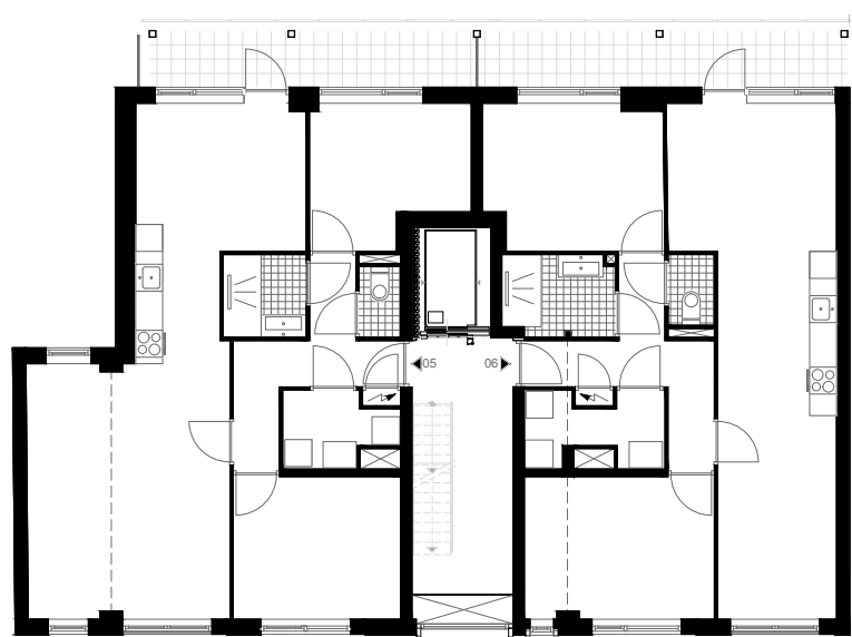
Tweede verdieping
