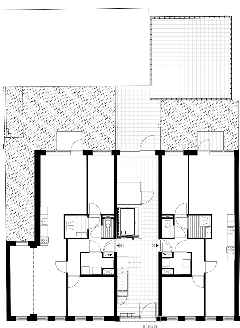
Begane grond
