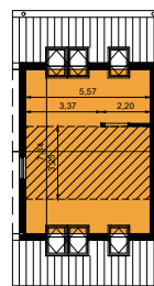
2e verdieping
