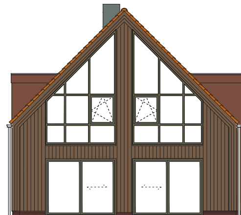
Zijgevel, optie 3: extra large + optie schuifpui
