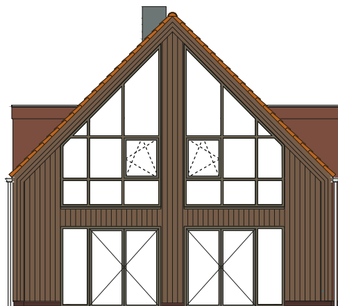
Zijgevel, optie 2: extra large
