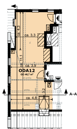
Tweede verdieping
