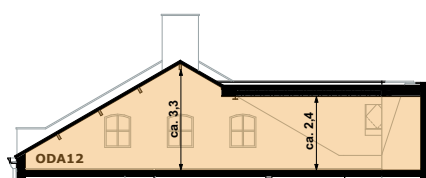
Doorsnede B-B
