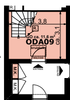
Begane grond
