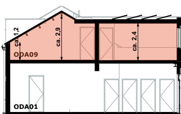
Doorsnede B-B
