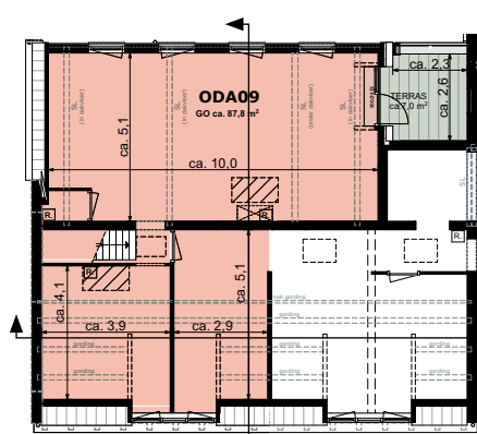
Eerste verdieping
