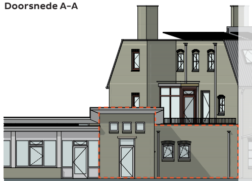
Linker parallelgevel
