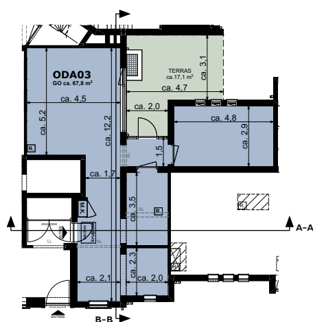
Begane grond
