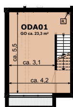
Souterrain
