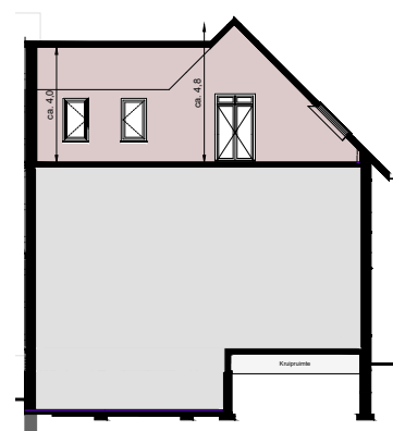
Doorsnede AA
