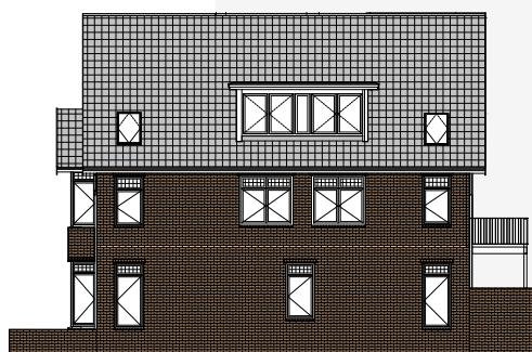
Zijgevel
