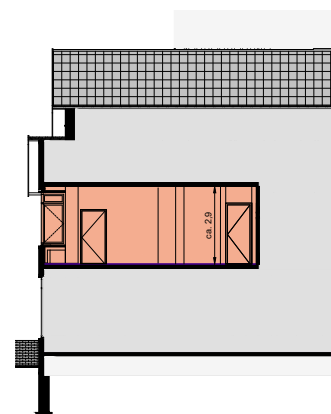
Doorsnede AA
